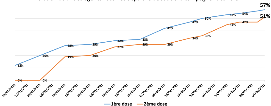
Evolution du % des agents vaccinés depuis le début de la campagne vaccinale
